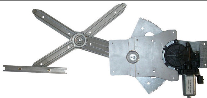
POWER WINDOW LEFT ALZACRISTALLI ELETTRICO SX
